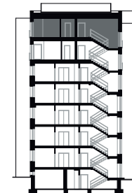
ŘEZ / PATRO
