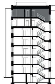
ŘEZ / PATRO
